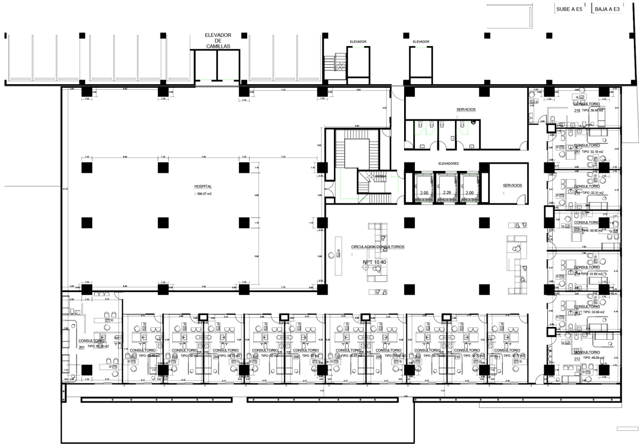
NIVEL 02
