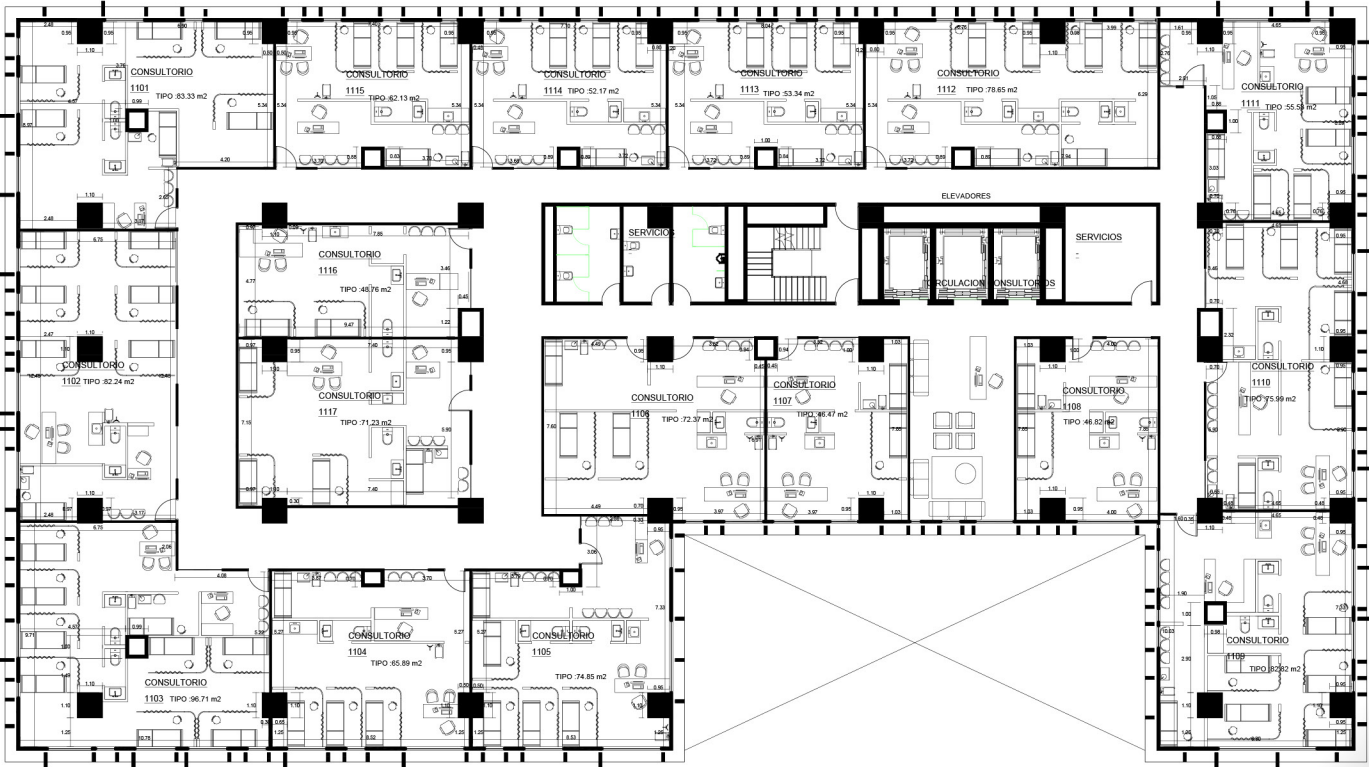
NIVEL 11
