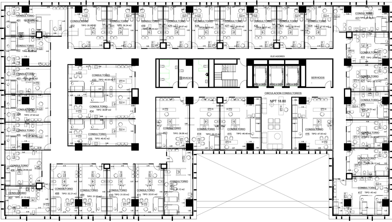
NIVELES 04, 05, 07, 08, 09 Y 10
